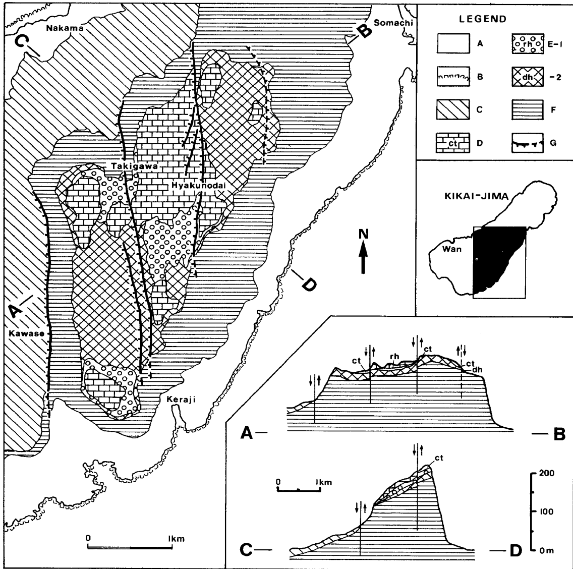
Fig. 40. Geological map of Kikai-jima for the Ryukyu Group. A : Raised Coral reefs and Recent alluvial deposits ; B : Recent coral reefs ; C : Wan Formation ; D : Takigawa Formation ; E : Hyakunodai Formation ; E-1 : Rhodolith limestone ; E-2 : Detrital limestone ; F : Shimajiri Group ; G : Fault.
