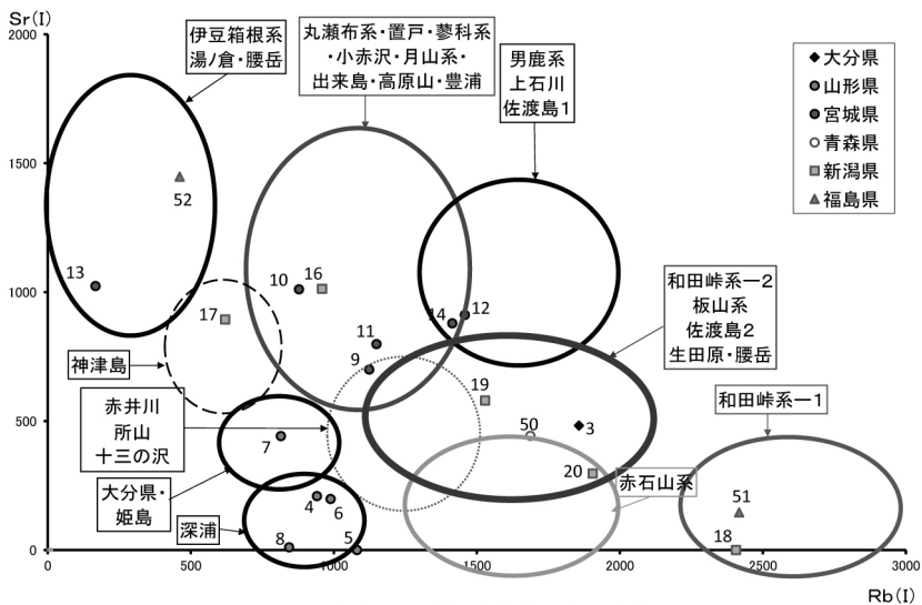
図6 日本の黒曜石 Rb-Sr 図
