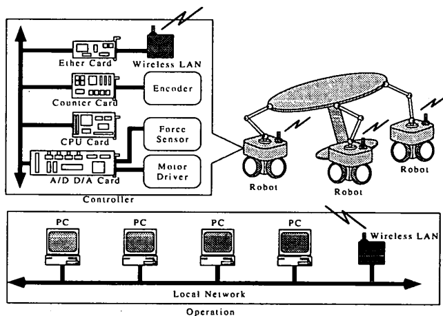
Fig. 4 Controller
