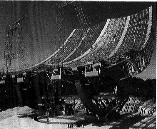
幅3.3メートル、高さ31メートル、約千平方メートルの巨大な開口面積。福島県相馬郡飯館村に設置された。
