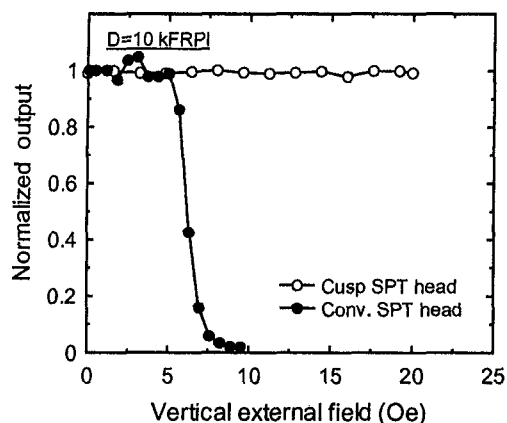
図 4. 外部浮遊磁界耐性
