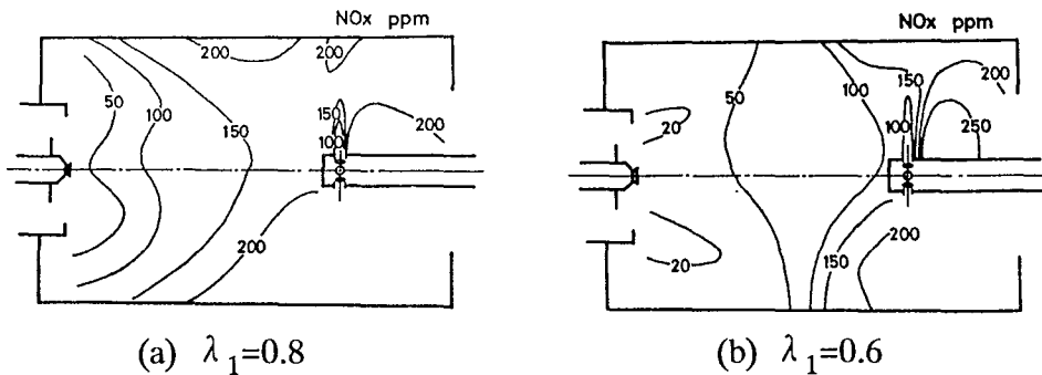
図2 NO x 濃度分布の一次空気比による変化 (含有窒素濃度=0.2wt%, 二次空気導入位置 Z s =200mm)
