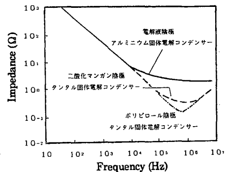
図2 インピーダンス-周波数特性
